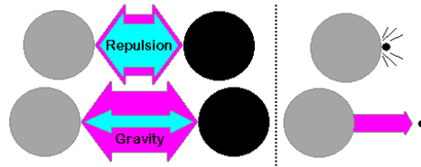
Illustration 2: force de répulsion gravitationnelle
