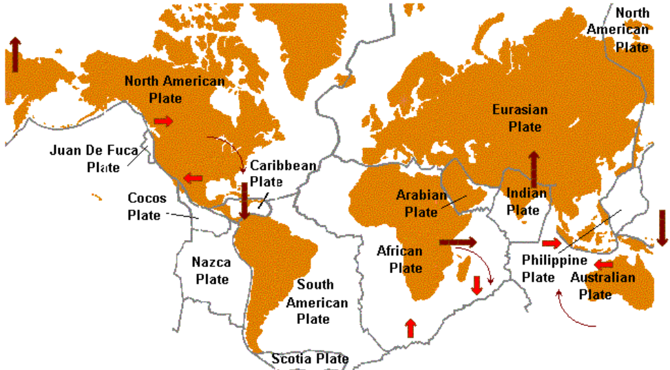
Figure 34: Plaques tectoniques mondiales
