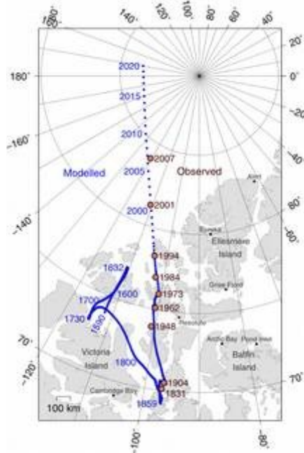
Figure 33: dérive pôle Nord magnétique
