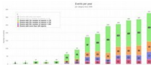
Figure 40: nombre météores entre 2006 et 2019
