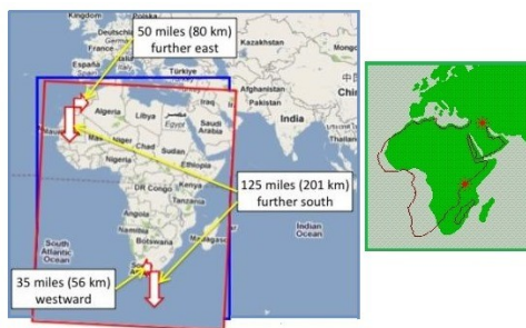
Figure 61: Rotation plaque tectonique africaine
