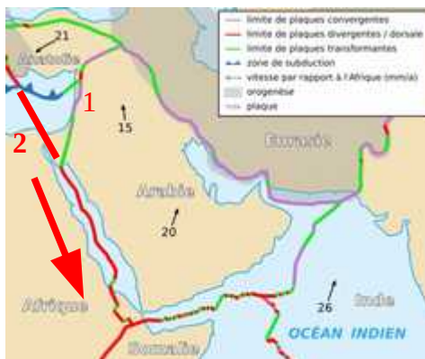
Figure 23: limites des plaques d'Islamie
