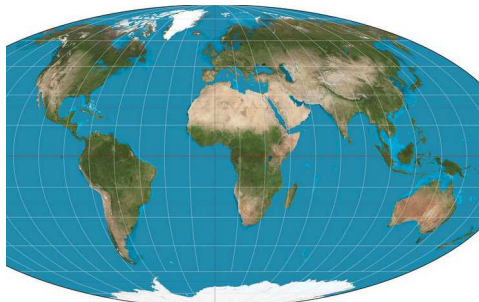
Figure 38: Projection elliptique (surfaces conservées)
