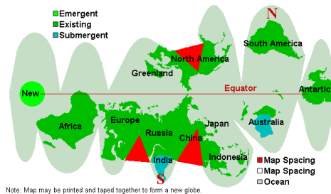
Figure 31: Terre 1 après PS2
