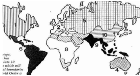
Figure 33: Club de Rome : découpe de la Terre en 1974
